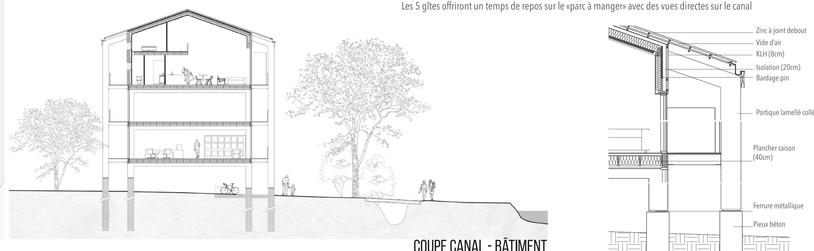
COUPE CANAL - BÂTIMENT
