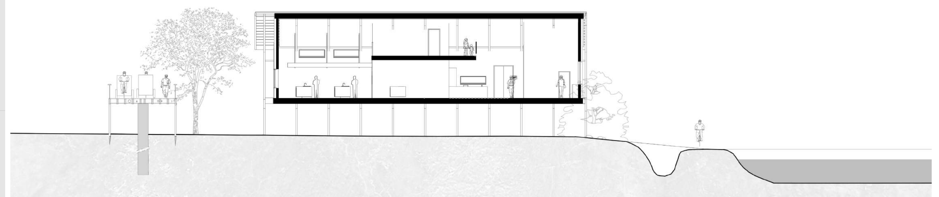
COUPE CANAL - LABORATOIRE
